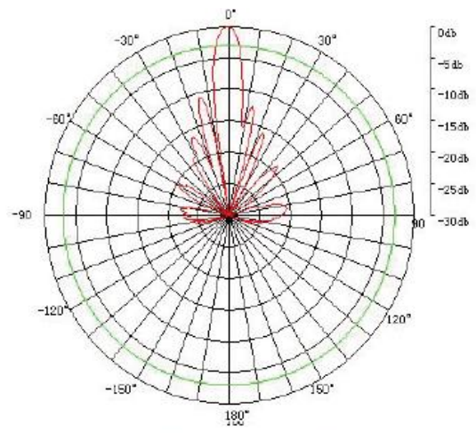
水平极化-垂直面
